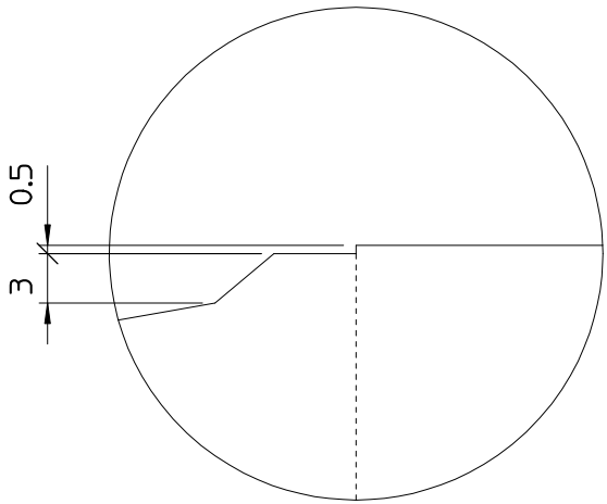
DETTAGLIO B
