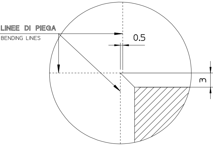
DETTAGLIO A
